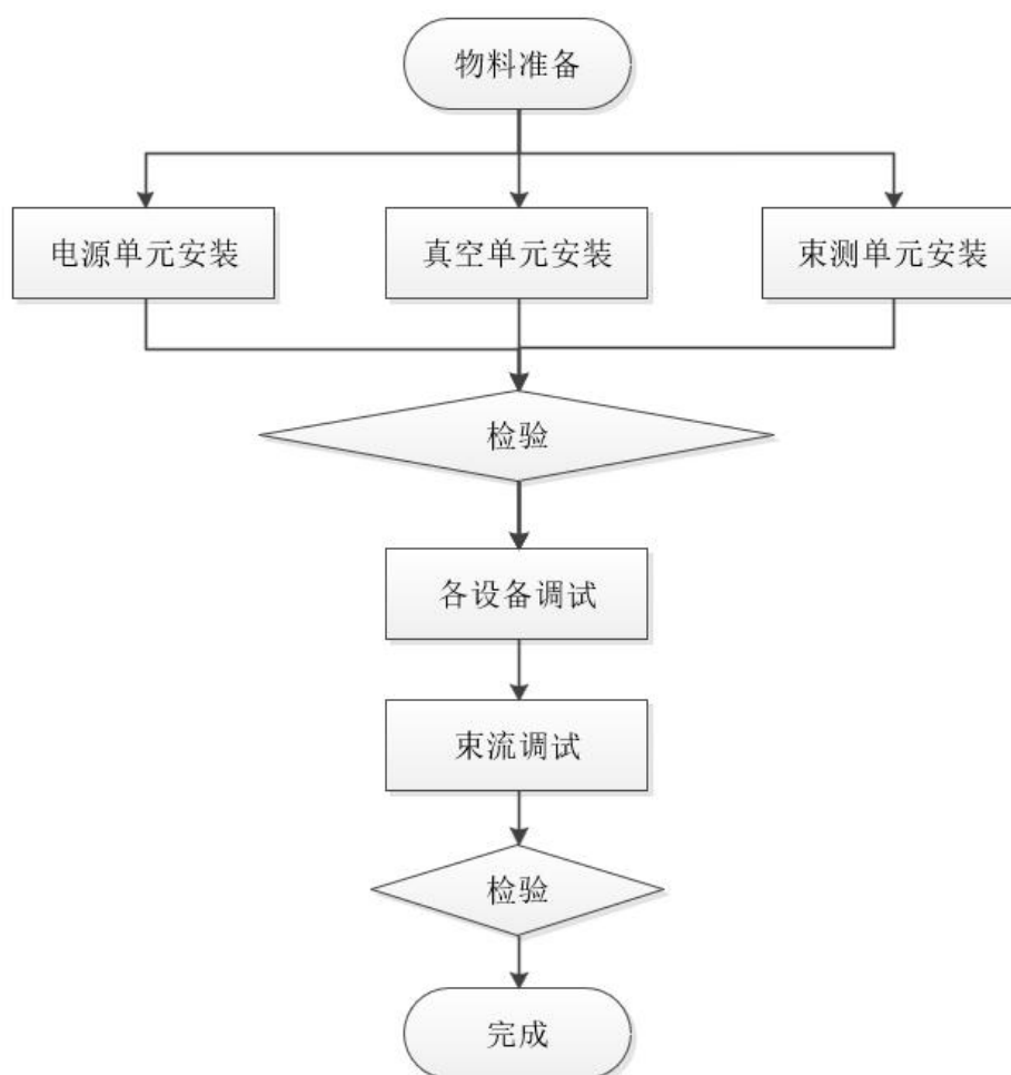
图 2 中能传输系统生产工艺流程图
