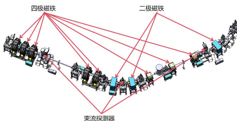
图 1 中能传输系统示意图
