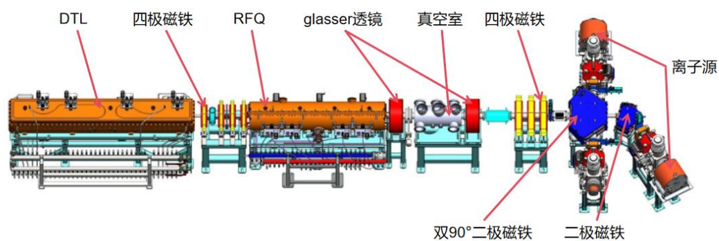
图 3 直线加速器示意图
