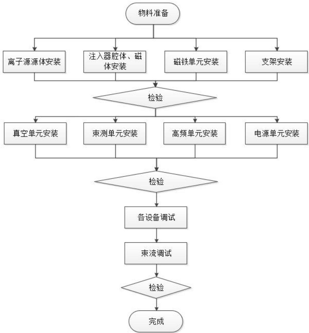
图 4 注入器系统生产工艺流程图
