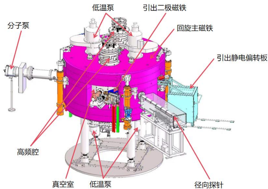
图 2 回旋加速器示意图
