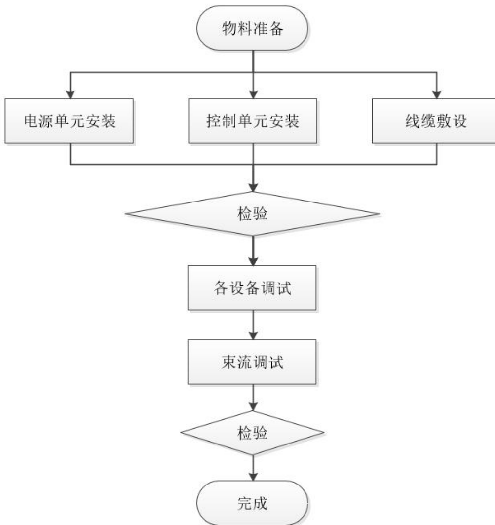
图 1 加速器辅助系统生产工艺流程图
