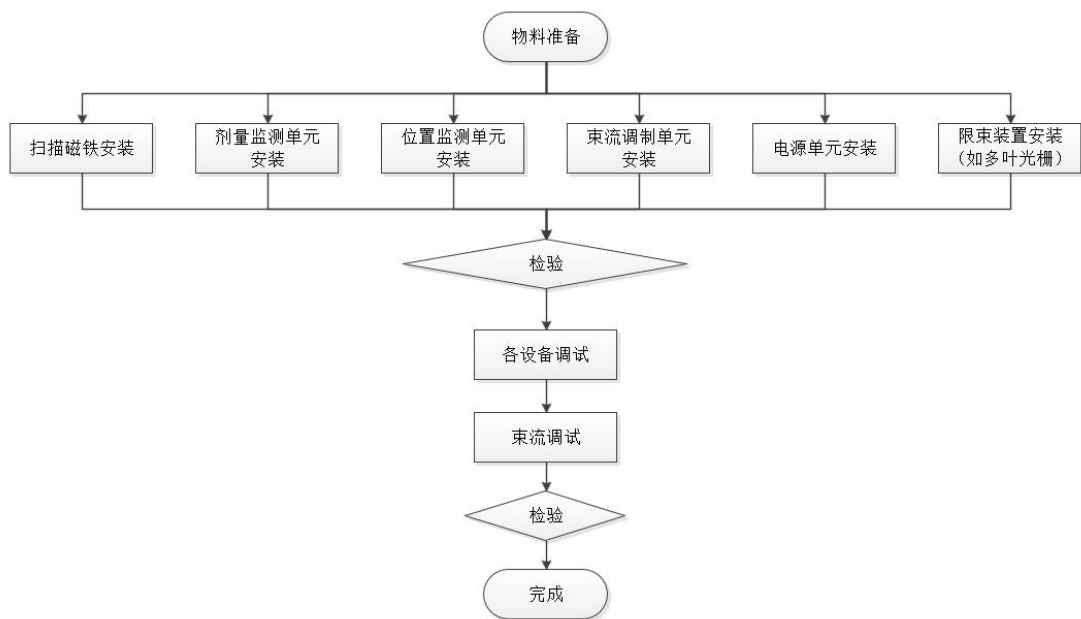
图2 被动式束流配送系统生产工艺流程图
