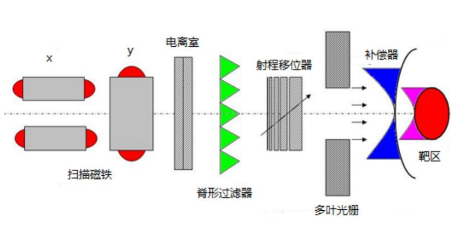
图 1 被动式束流配送系统示意图
