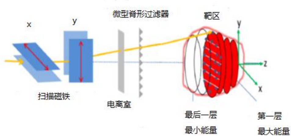
图 1 主动式束流配送系统示意图
