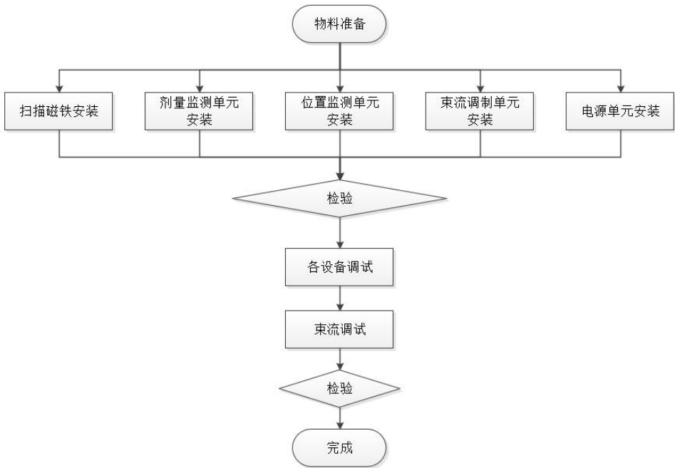
图 2 主动式束流配送系统生产工艺流程图
