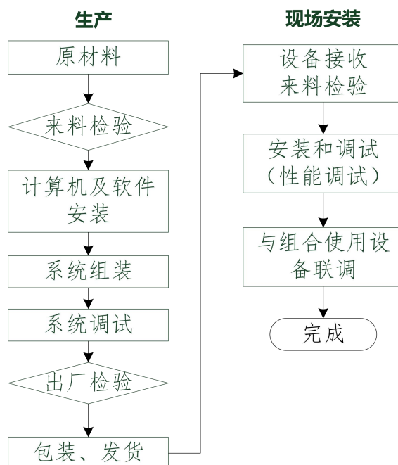
图 1 呼吸门控与运动管理系统生产工艺流程图
